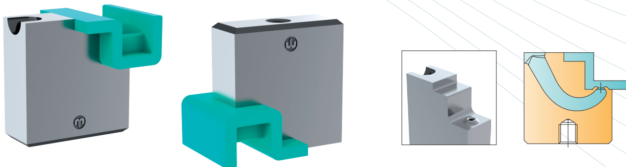
TGLL low contour step / TGLL perfil inferior / TGLL profil bas
